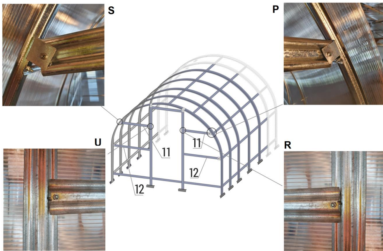
Obr. 5 (detaily S a P jsou pohled zvenku konstrukce, detaily U a R pohled zevnitř konstrukce)
